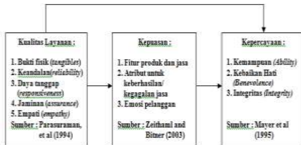
Gambar 1 Kerangka Teori
