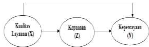
Gambar 2 Kerangka konsep
